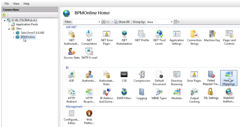
Рис. 461 — Переход в Handler Mappings
