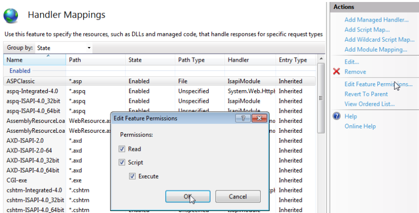
Рис. 462 — Проверка необходимых параметров в окне [Edit Feature Permissions]
