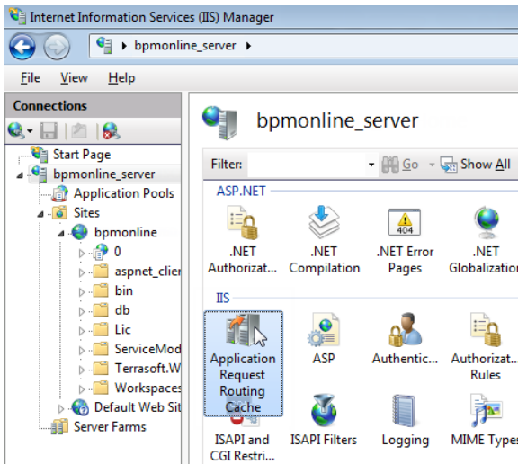
Рис. 242 — Переход к настройке [Application Request Routing]
