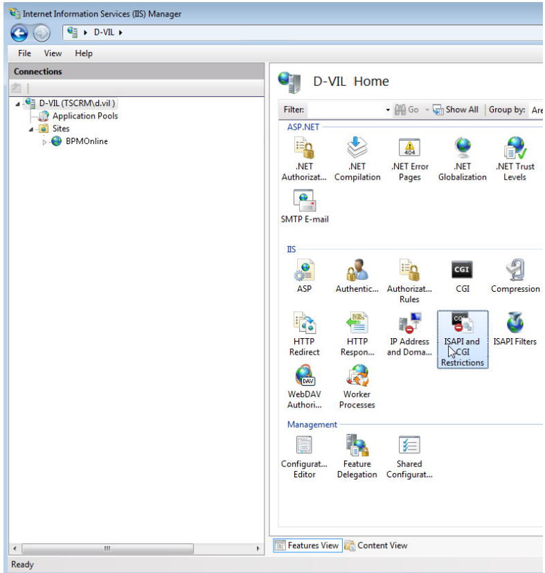
Рис. 459 — Переход в ISAPI and CGI Restrictions
