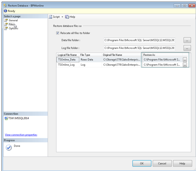
Рис. 447 — Указание названий файлов и путей размещения файлов S_Data.mdf и TS_Log.ldf.
