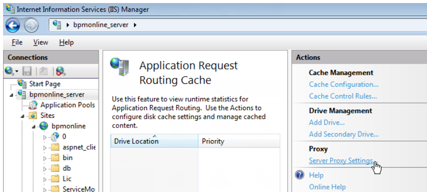
Рис. 243 — Переход к настройкам прокси
