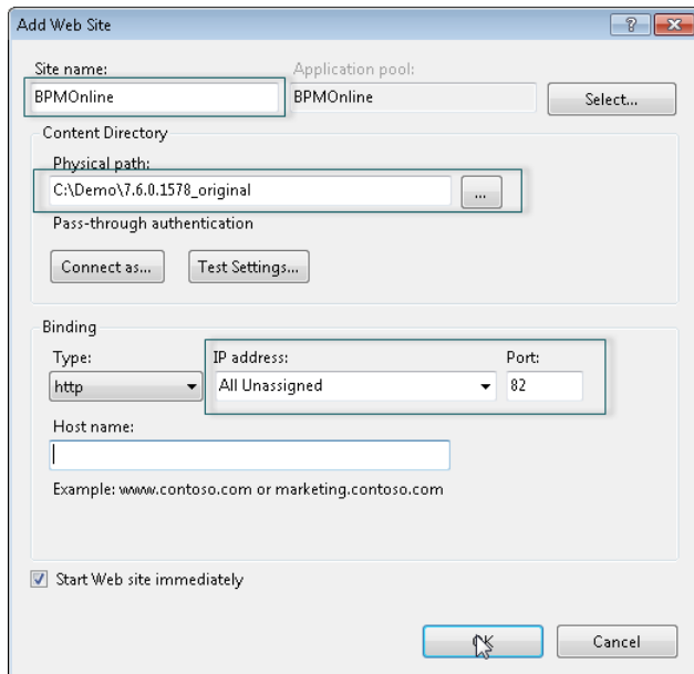
Рис. 455 — Окно параметров нового сайта
