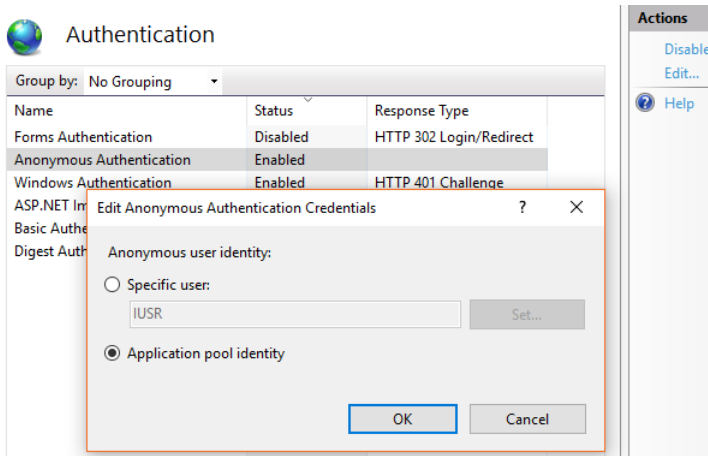
Рис. 425 — Указание пользователя для анонимной аутентификации в настройках IIS
