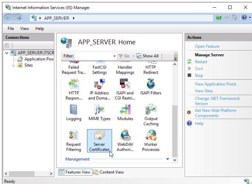
Рис. 464 — Выбор детали [Server Certificates]
